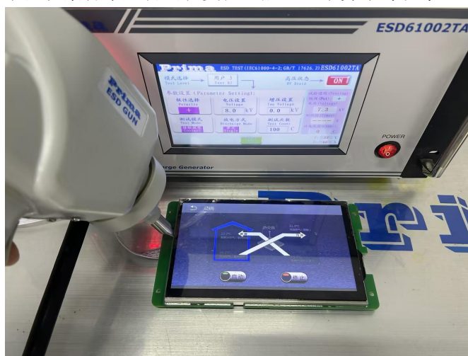
图 5-2 ESD 测试图
